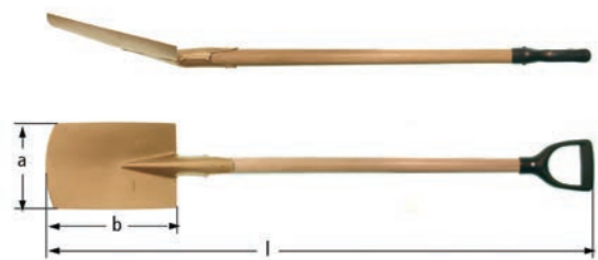
D型柄边铲 Edging spade with D-handle - Spaten mit D-stiel - Béche, manche à poignée
