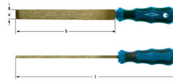
扁刮刀 Scraper, flat - Flachscher - Grattoir de mécanicien
